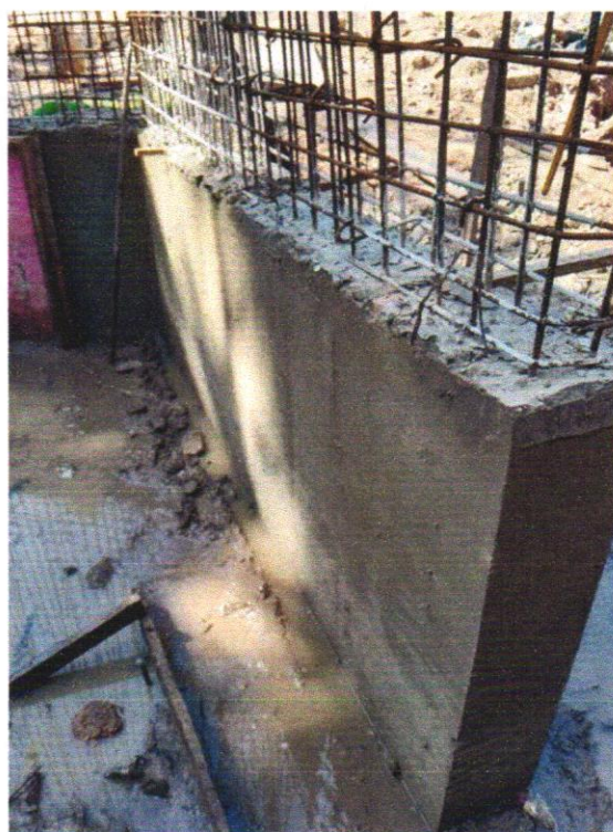
Concretagem de Ancoramento de Estrutura
